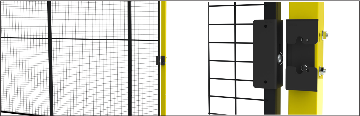
T10-30 Elementy mocujące, drzwi przesuwne MGB Euchner, prawe/lewe.
