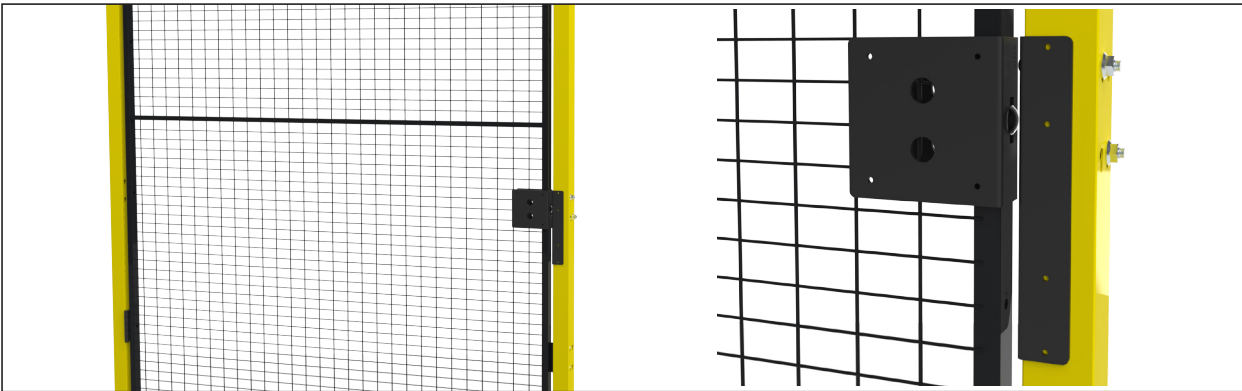
T10-32 Elementy mocujące, drzwi uchylne Schmersal AZM200, prawe/lewe.
