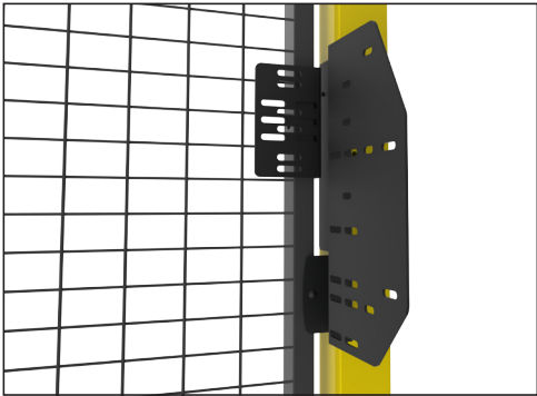
T10-12 Komplet elementów mocujących do wyłącznika bezpieczeństwa i klucza, drzwi uchylne, prawe/lewe, Euchner.
