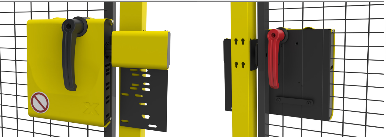
X-Lock X-Lock to wszechstronny system zamków pasujący do wszystkich naszych serii produktów zapobiegających wypadkom. Wykorzystując zamek X-Lock i zestaw drzwiowy, można przekształcić każdy panel służący do zapobiegania wypadkom w drzwi z funkcją bezpiecznego blokowania. Zamek X-Lock wyposażony jest w mechaniczny trzpień utrzymujący drzwi uchylne i przesuwne w położeniu
