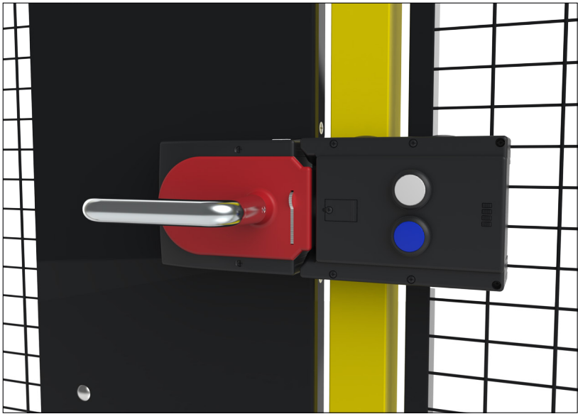
MGB firmy Euchner MGB (Multifunctional Gate Box) to wyjątkowy system blokad wewnętrznych i blokad osłon do ochrony drzwiczek zabezpieczających maszyn i systemów. Cztery diody LED wskazują stan zamka. Zamek wyposażony jest w inteligentny trzpień, którego położenie rejestrowane jest przełącznikiem RFID o unikalnym kodzie. Zapobiega to manipulowaniu przy zamku, przy czym MGB spełnia normy EN ISO 13849-1 / SIL 3 zgodnie z EN 62061.
