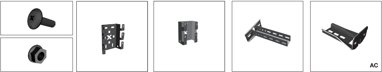
Śruba X61 M8x27 Nr elementu 2761 40 sztuk Obejma X10 Nr elementu 2710-1 Miniobejma X10 Nr elementu 2710-2 Wysięgnik X11 Nr elementu 2711-240 Wysięgnik X14 Nr elementu 2714-280
